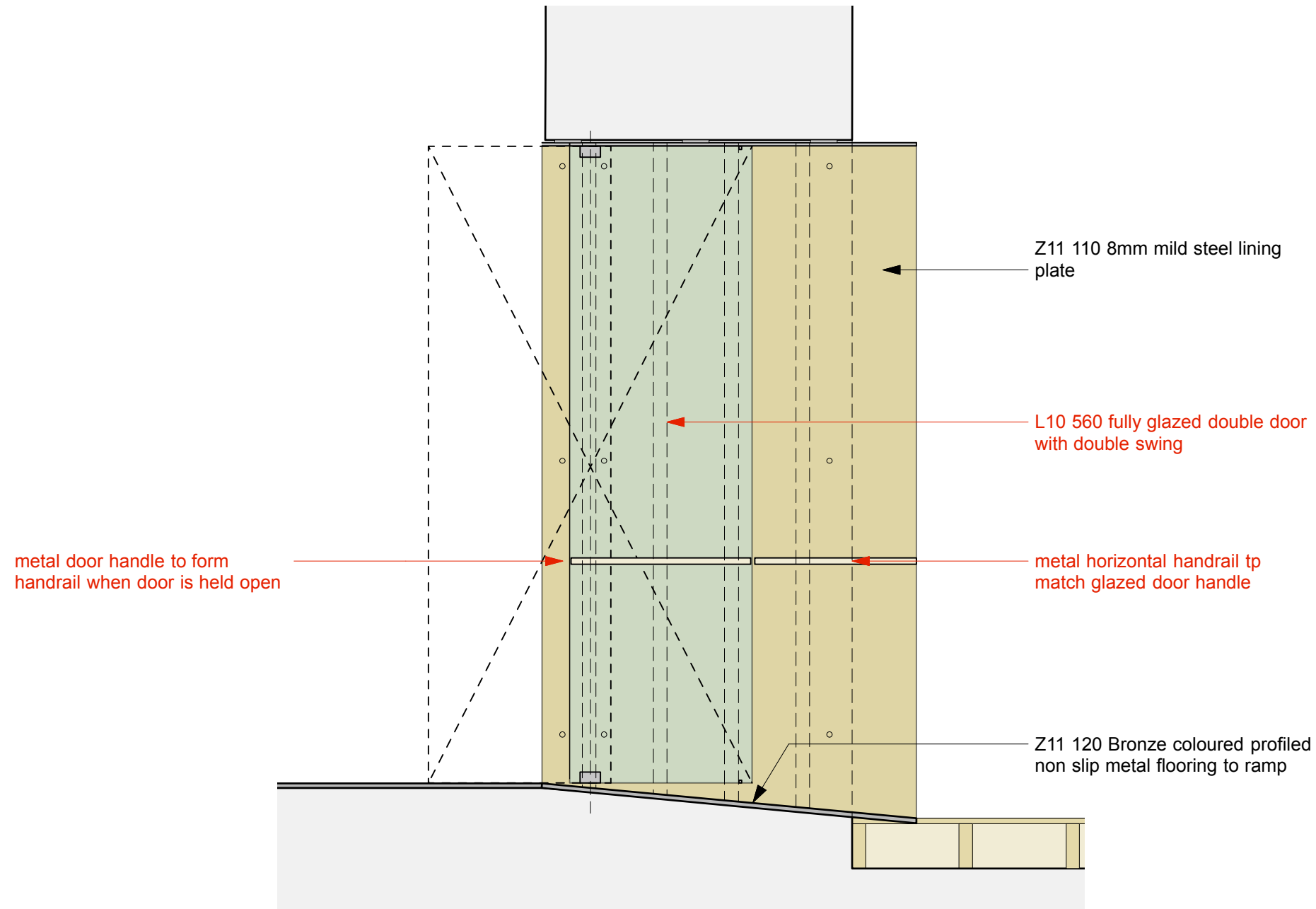
1 Section Scale: 1:20
