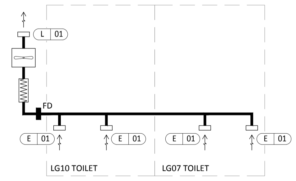
VENTILATION SCHEMATIC N.T.S.
